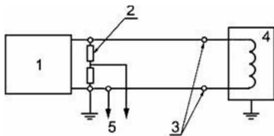
1 - генератор импульсов; 2 - делитель напряжения; 3 - соединительные контактные зажимы; 4 - испытуемое балластное устройство; 5 - контактные зажимы для присоединения электронного осциллографа Рисунок 5 - Электрическая схема установки для испытаний импульсом высокого напряжения
